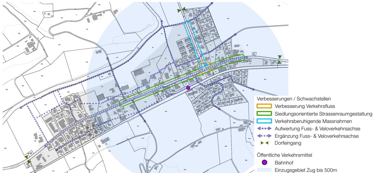
Abb. 11: Übersicht über die Erschliessung, Schwachstellen und Abschnitte mit Massnahmen
