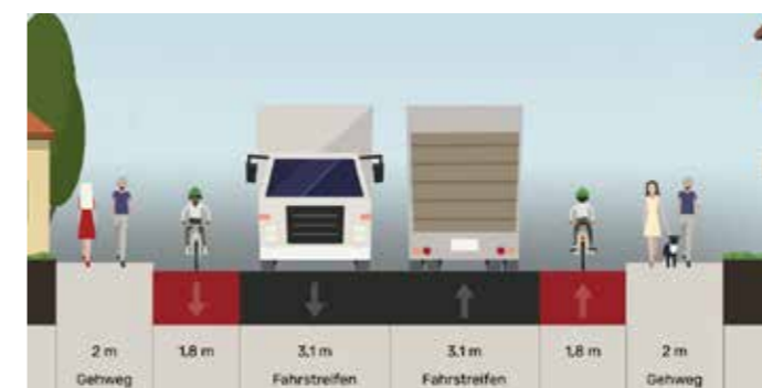
Abbildung 3: Mögliche neue Gestaltung des Strassenraums in der Variante Null+/ Neugestaltung – Zentrum Schötz mit Radstreifen.
