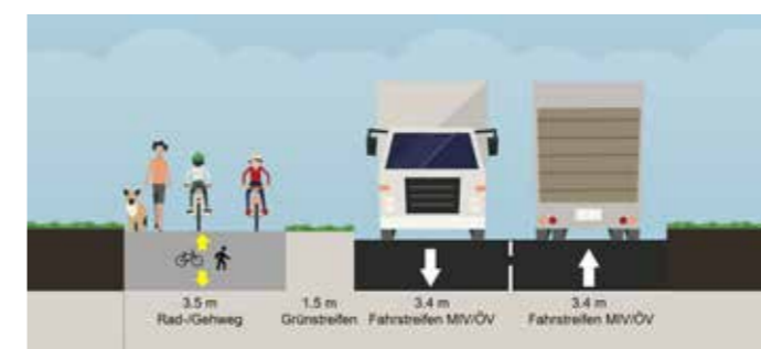
Abbildung 4: Mögliche neue Gestaltung des Strassenraums in der Variante Null+/ Neugestaltung – einseitiger Rad-Gehweg zwischen Schötz und Alberswil.
